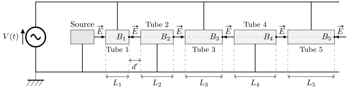
FIGURE 1 – Accélérateur de Wideröe
